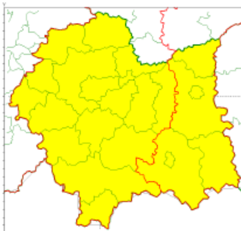
Opady marznące 2021-02-18 13:55
